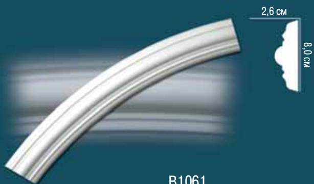
B1061 внутренний \varnothing 89,0 см внешний \varnothing 105,0 см
