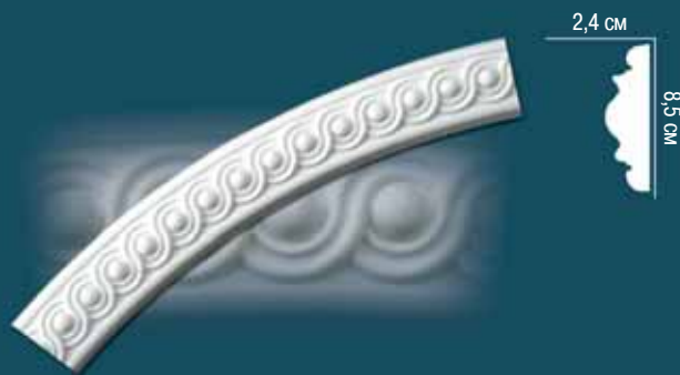
B1063 внутренний \varnothing 87,5 см внешний \varnothing 104,5 см
